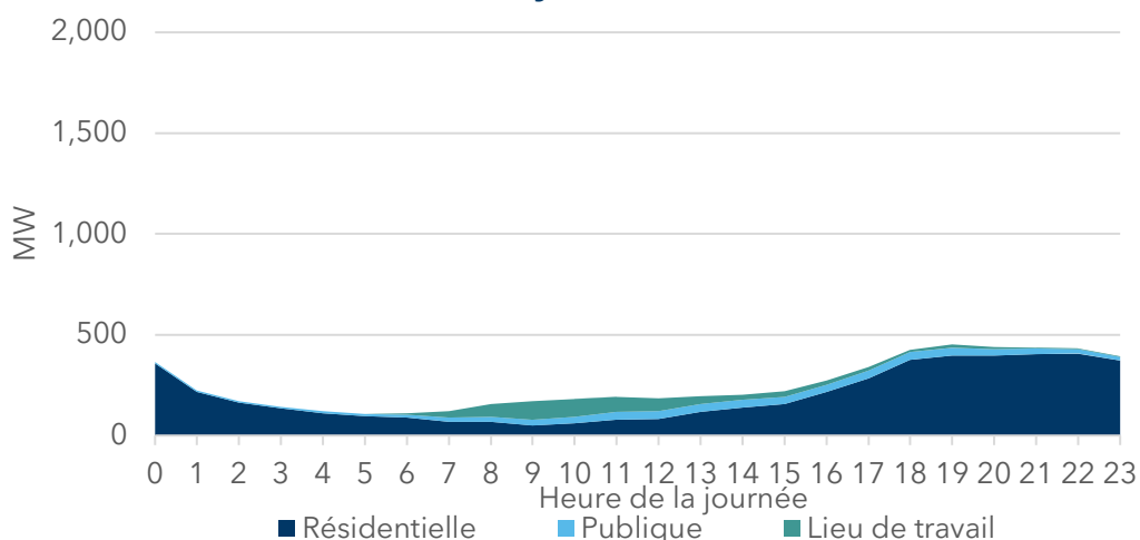
Graphique 26. Demande liée à la recharge des VZE lors de la journée de pointe estivale en 2040, croissance moyenne, Manitoba
