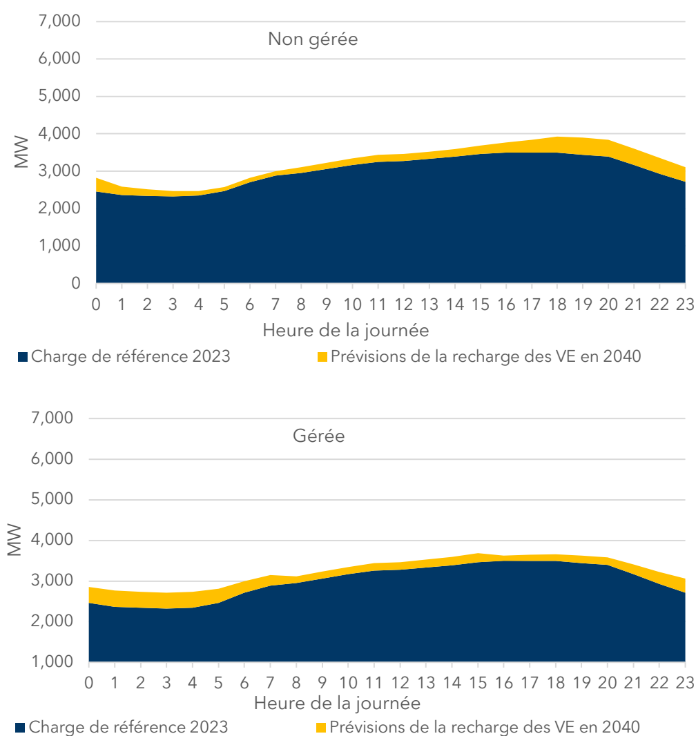
Graphique 28. Potentiel de la gestion de la recharge, journée de pointe estivale, croissance moyenne, Manitoba
