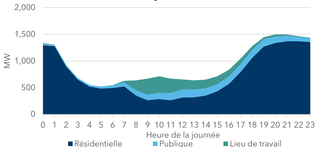
Graphique 27. Demande liée à la recharge des VZE lors de la journée de pointe hivernale en 2040, croissance moyenne, Manitoba
