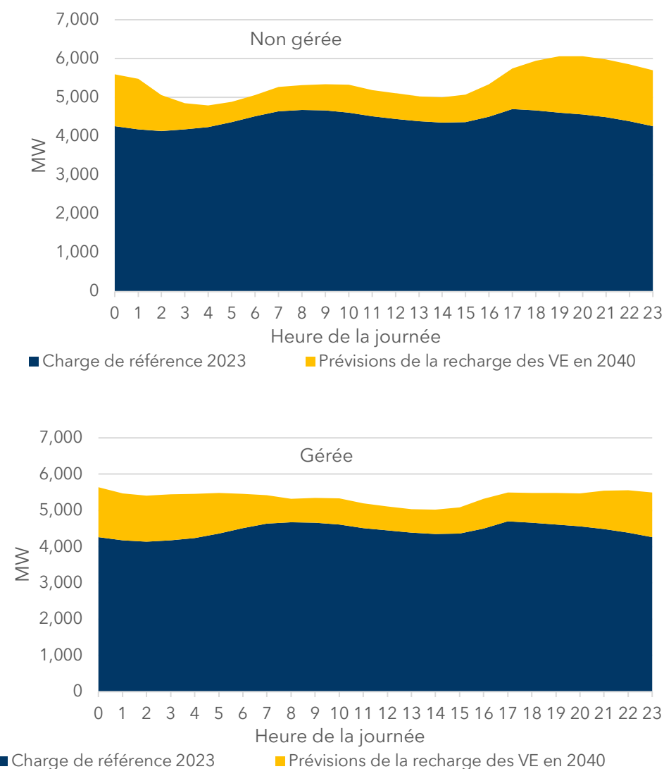
Graphique 29. Potentiel de la recharge gérée, journée de pointe hivernale, croissance moyenne, MB
