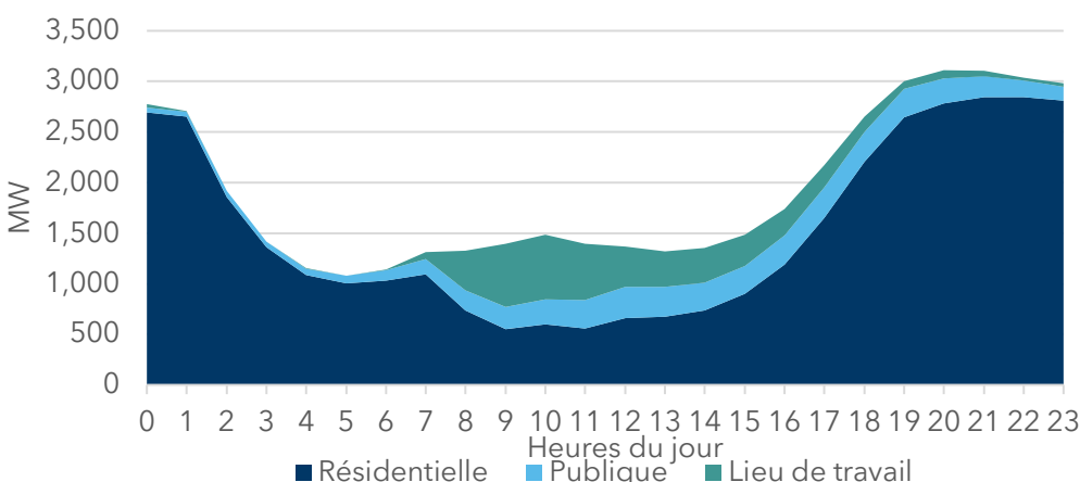
Graphique 27. Demande liée à la recharge des VZE lors de la journée de pointe hivernale en 2040, croissance moyenne, AB
