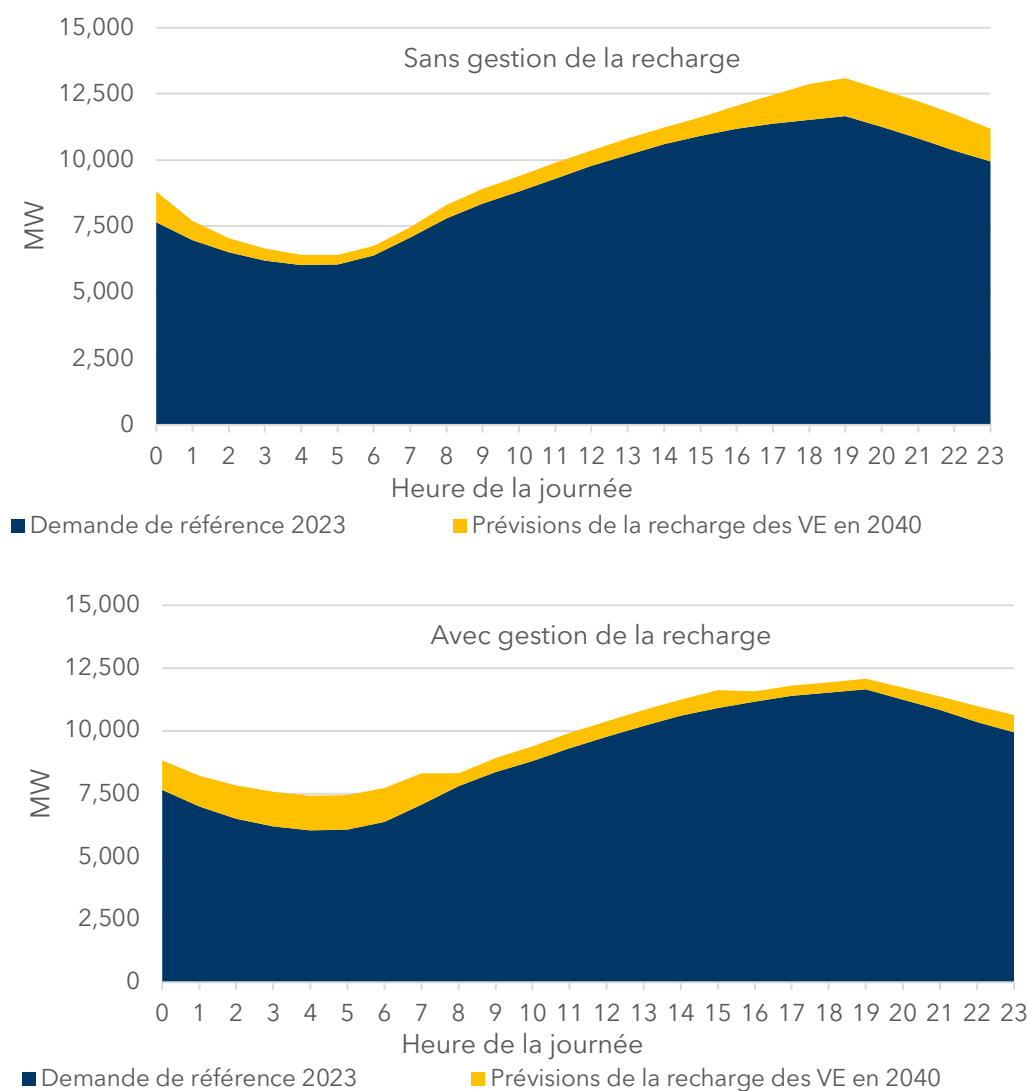
Graphique 28. Potentiel de la gestion de la recharge, journée de pointe estivale, croissance moyenne, AB
