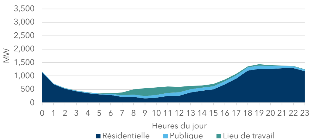
Graphique 26. Demande liée à la recharge des VZE lors de la journée de pointe estivale en 2040, croissance moyenne, AB
