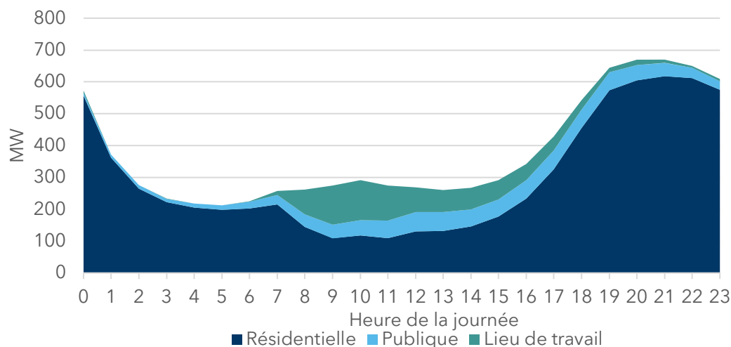
Graphique 27. Demande liée à la recharge des VZE lors de la journée de pointe hivernale en 2040, croissance moyenne, Nouveau-Brunswick
