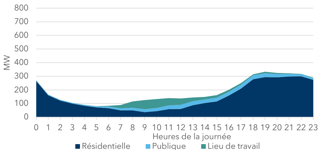
Graphique 26. Demande liée à la recharge des VZE lors de la journée de pointe estivale en 2040, croissance moyenne, Nouveau-Brunswick
