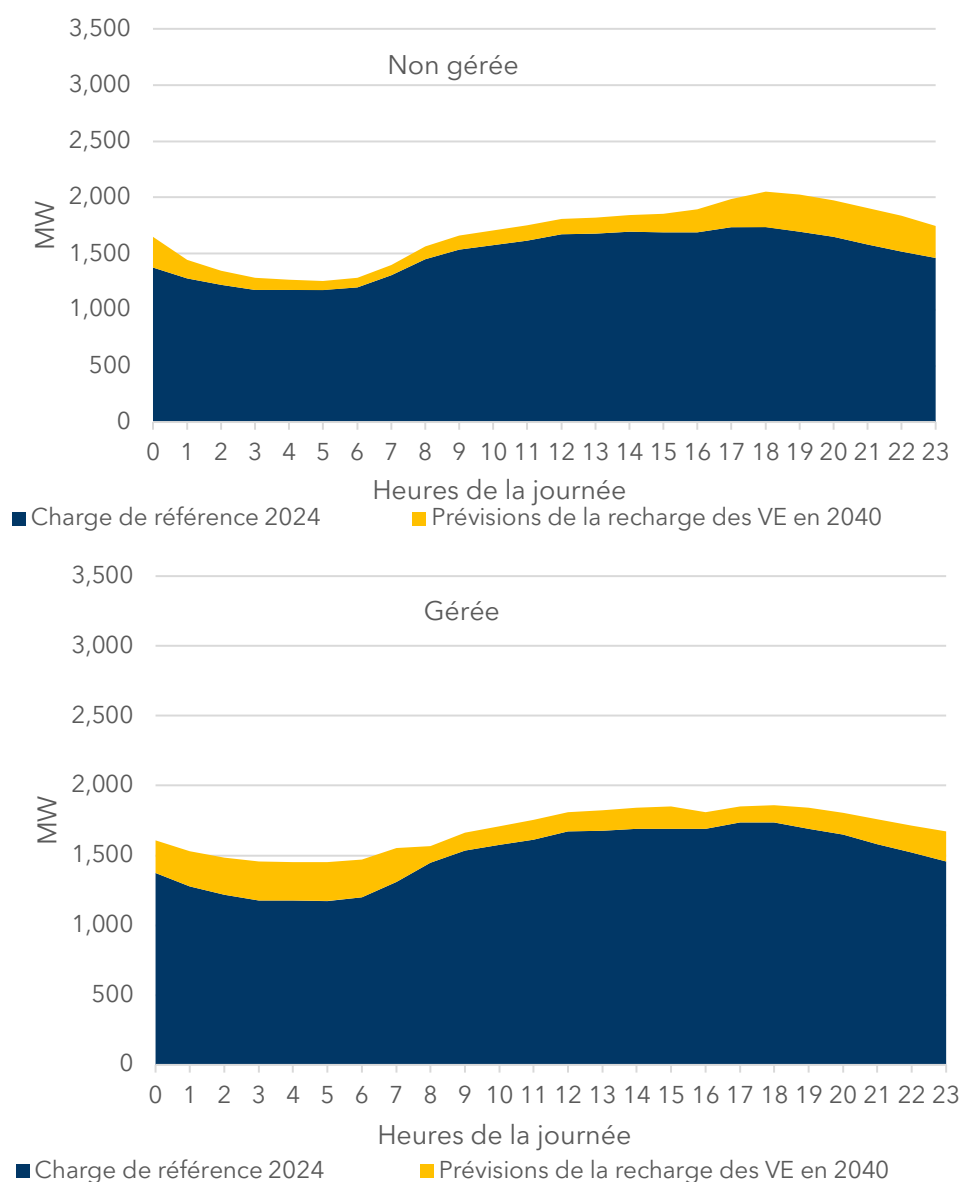
Graphique 28. Potentiel de la gestion de la recharge, journée de pointe estivale, croissance moyenne, Nouveau-Brunswick
